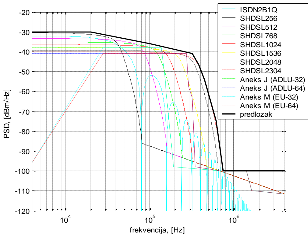
Slika 5.6.3 Frekvencijski predložak za odlazni smjer prijenosa (pretplatničke linije srednje duljine).
